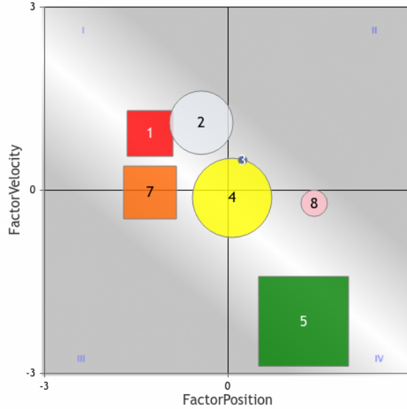
OptixPlot-SURFDIST
